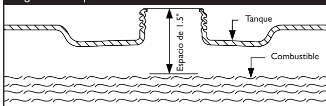
Figura 13 - Espacio de Combustible
