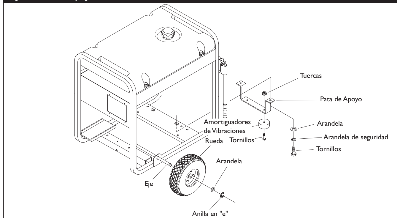
Figura 12 — Instale el Juego de Ruedas
