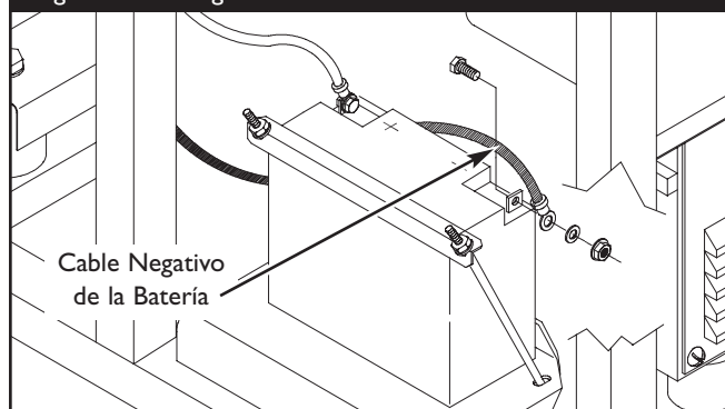
Figura 11 — Negativo Alambre las Conexiones
